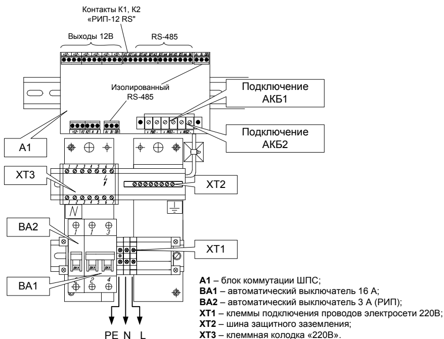
Рисунок 2 Схема расположения основных элементов «ШПС»
