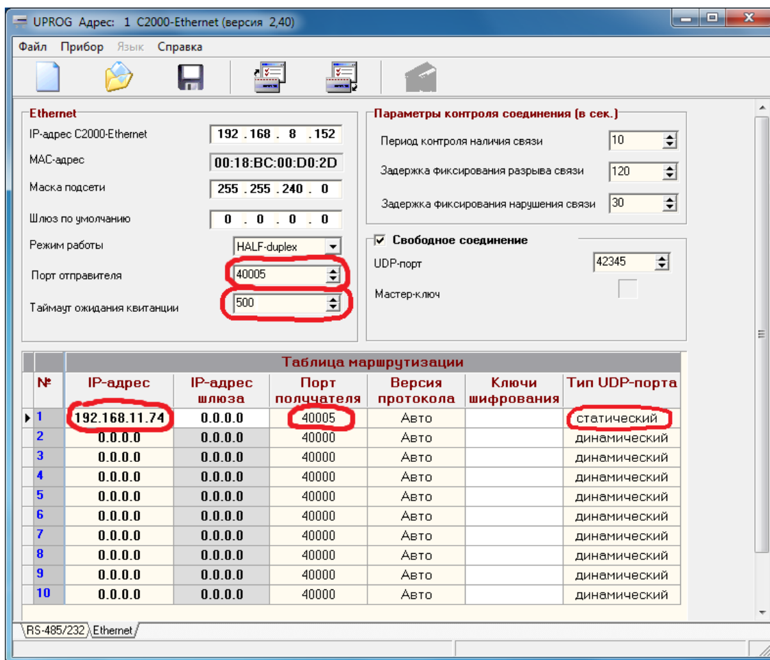
Рис.6. Параметры настройки C2000-Ethernet, страница Ethernet.
